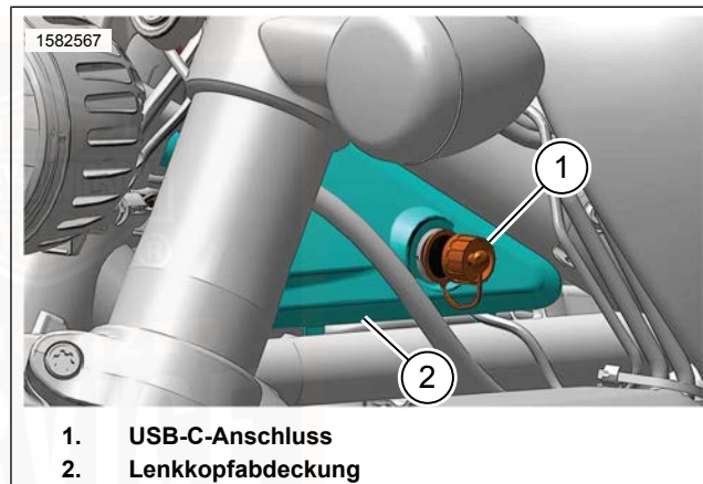
Abbildung 47. USB-C-Anschluss
