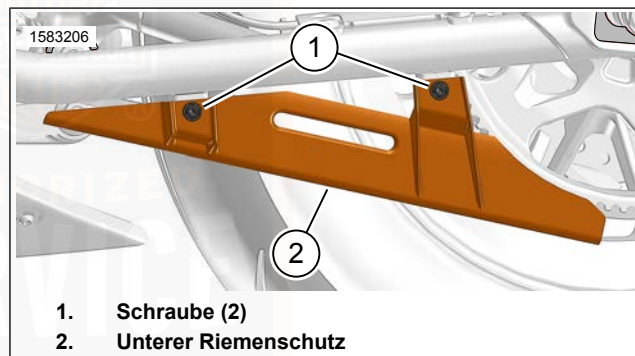
Abbildung 64. Unterer Riemenchutz
