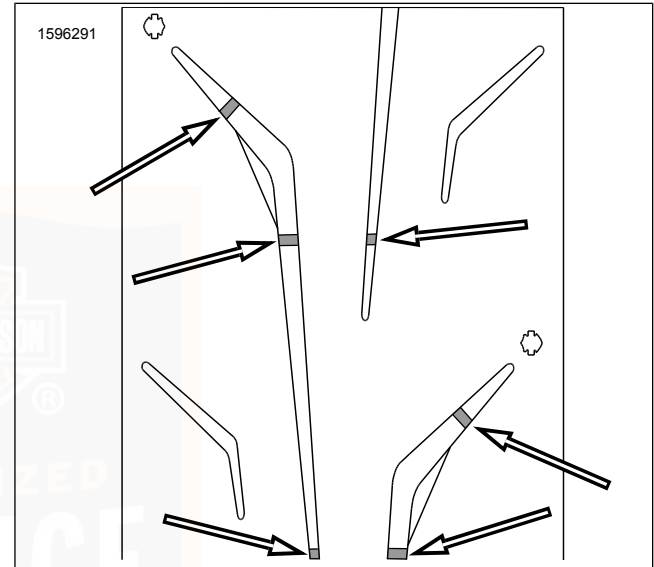
Abbildung 15. Dunlop-Reifen, Aussehen der Profilvererschleißanzeigen
