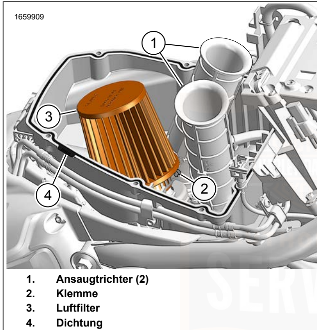
Abbildung 74. Luftfilterwartung
