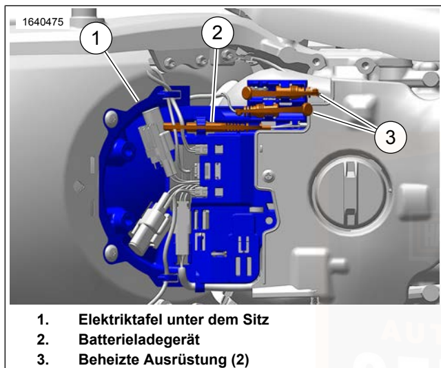
Abbildung 49. Unter dem Sitz (Kraftstofftank unter dem Sitz)
