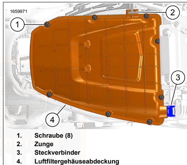
Abbildung 73. Luftfiltergehäuseabdeckung
