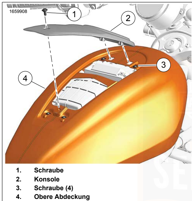
Abbildung 72. Obere Abdeckung
