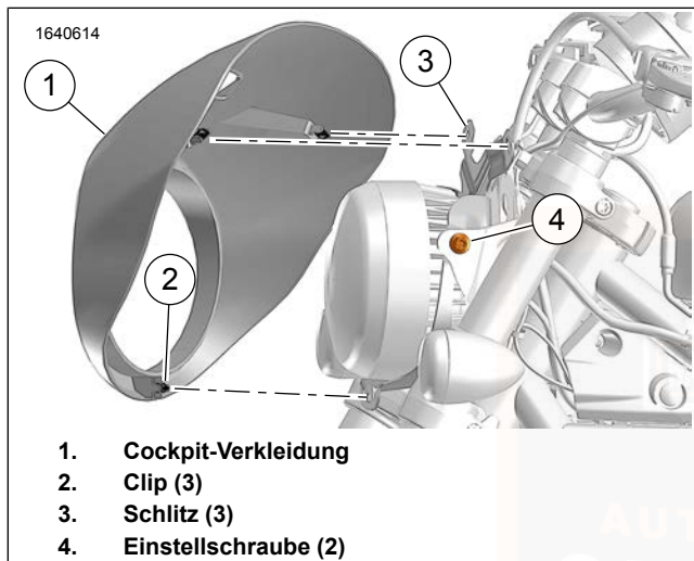
Abbildung 94. Scheinwerfereinstellschraube: RH975S (linke Seite abgebildet)
