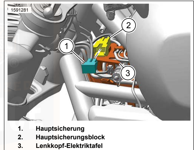
Abbildung 98. Lage der Hauptsicherung (RH1250S)
