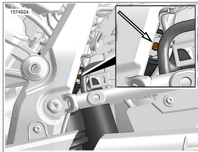
Abbildung 20. Kompressionseinsteller
